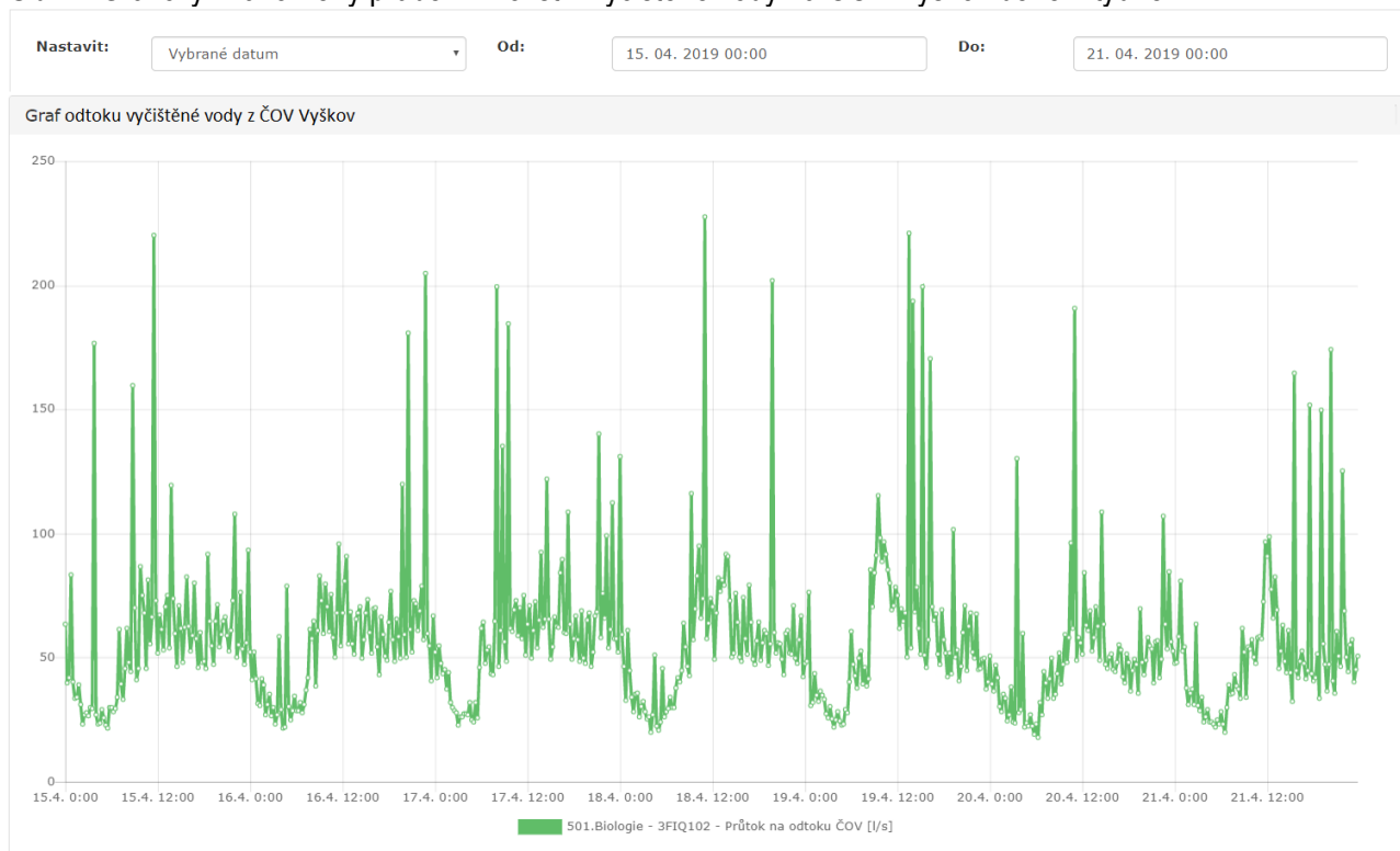
Obr. 2 Graficky znázorněný průběh množství vyčištěné vody na ČOV Vyškov během týdne
