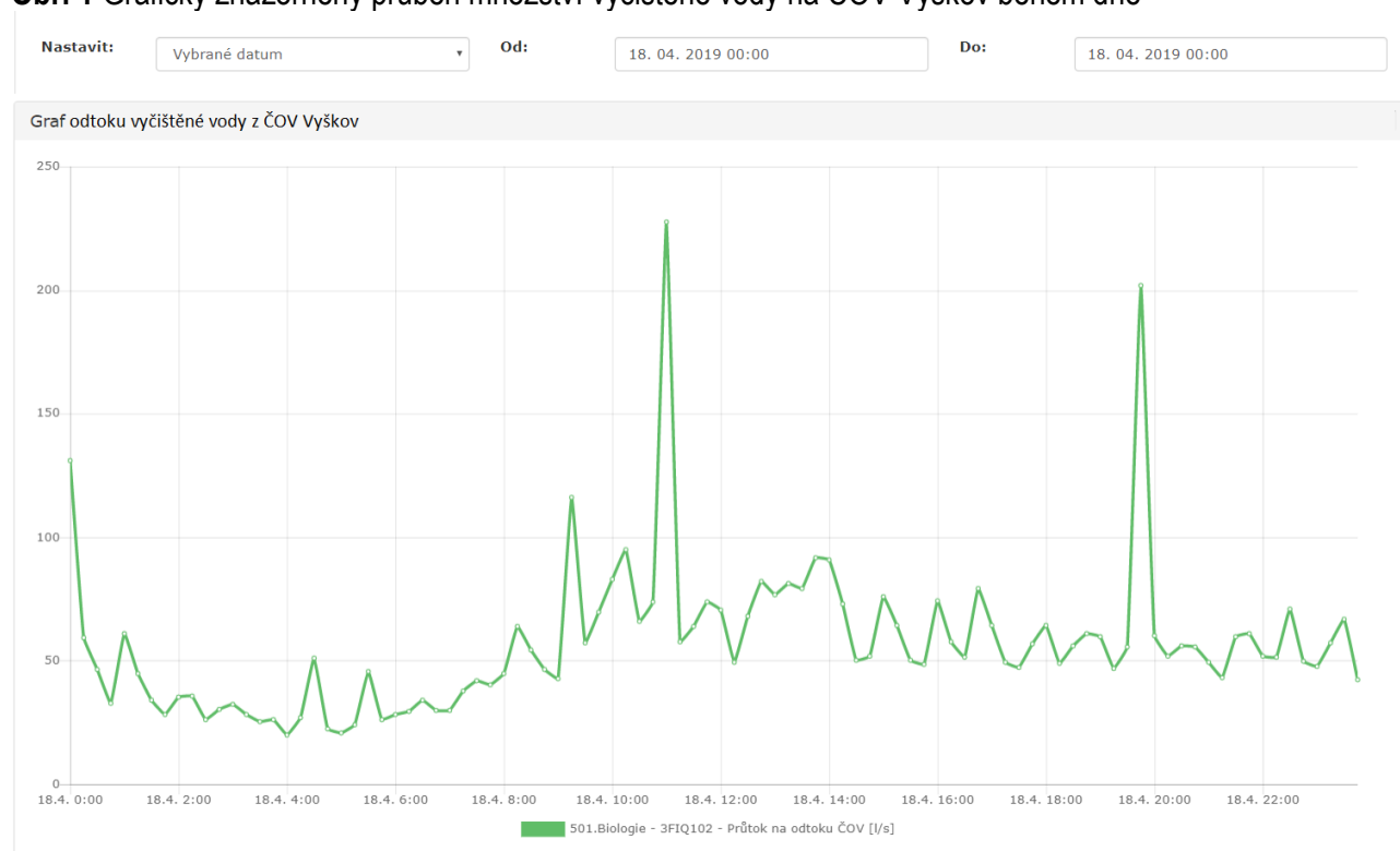
Obr. 1 Graficky znázorněný průběh množství vyčištěné vody na ČOV Vyškov během dne
